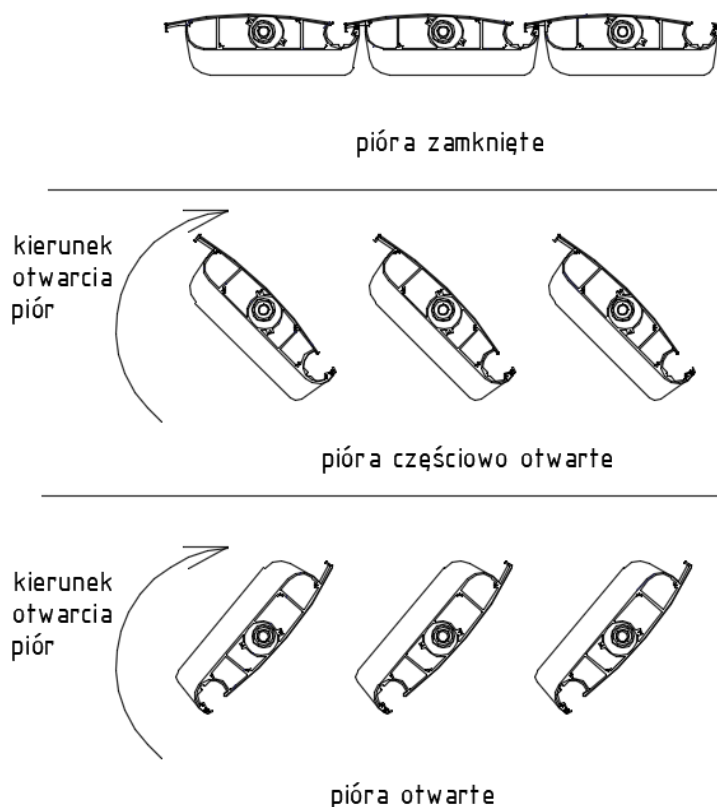
Rys. 3. Standardowe ustawienie kierunku otwierania piór w Pergoli SB400PRO
